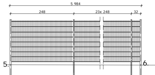
odcinek 3. -4. l = 59,84m
