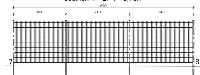
odcinek 1. -2. l = 6,90m
