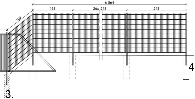
odcinek 5. -6. l = 69,67m
