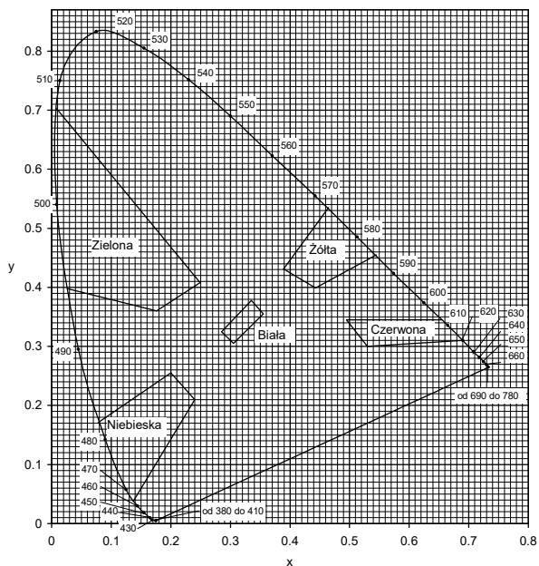
Rys. 3. Granice barw bialej, żoltej, czerwonej, niebieskiej i zielonej oznakowania
