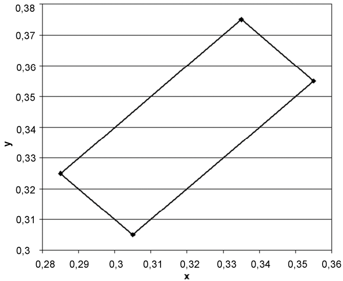
Rys. 1. Współrzędne chromatycyjnosc x,y dla barwy bialej oznakowania
